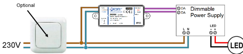
Typisches Schaltbild Typical connection scheme
