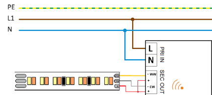
Typisches Schaltbild Typical connection scheme
